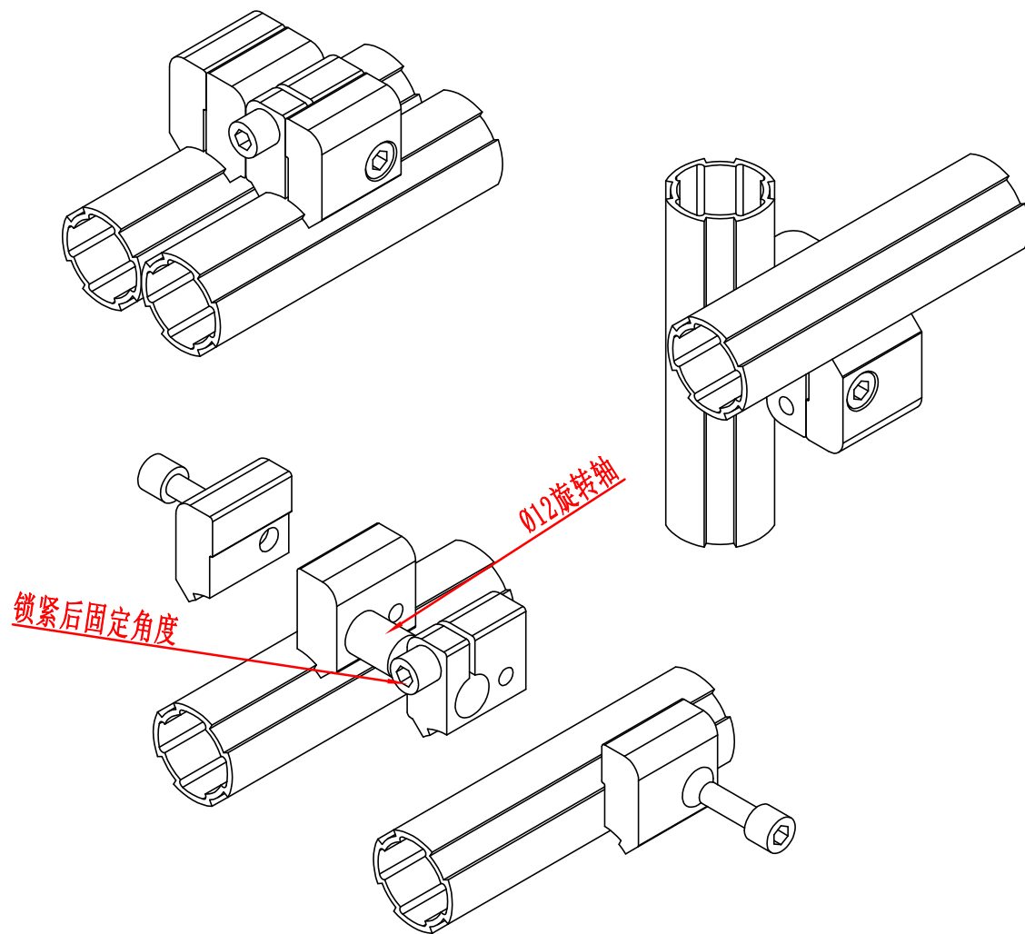
安装示意图
